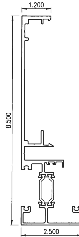
21 SUN-8119 SPLIT MULLION Scale: 6" = 1'-0"
