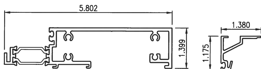
5 SUN-6316 FACE CAP Scale: 6" = 1'-0"
