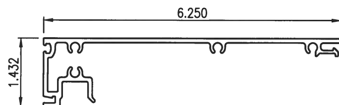
14 SUN-8288 SILL Scale: 6" = 1'-0"
