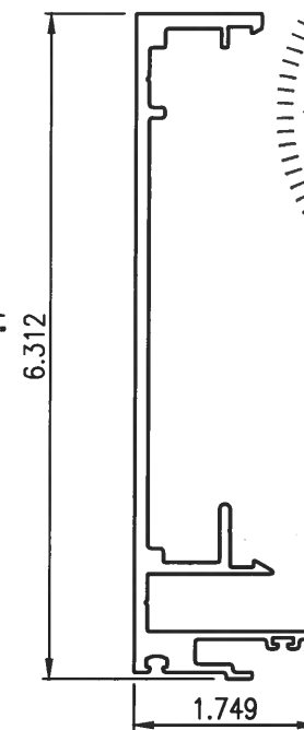
27 SUN-8209 B.G. SPLIT MULLION Scale: 6" = 1'-0"
