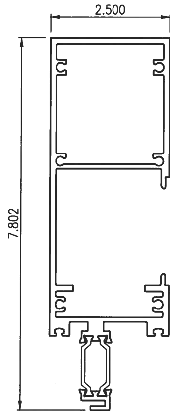
25 SUN-8120 JAMB Scale: 6" = 1'-0"
