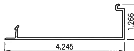
6 SUN-8221 HEAD Scale: 6" = 1'-0"
