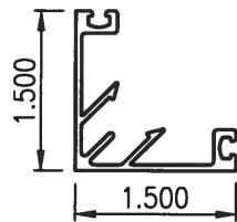
29 SUN-7064 90° FACECAP Scale: 6" = 1'-0"
