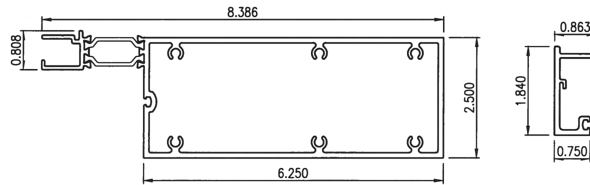
3 SUN-8321 HEAD Scale: 6" = 1'-0"
