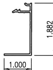
33 SUN-8290 SILL CLOSURE Scale: 6" = 1'-0"
