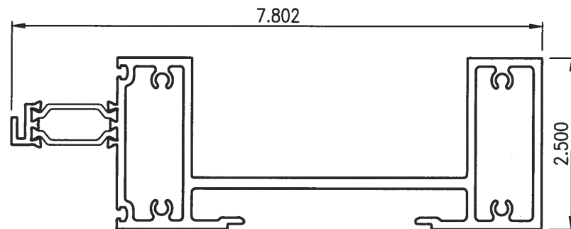
6 SUN-8221 HEAD Scale: 6" = 1'-0"
