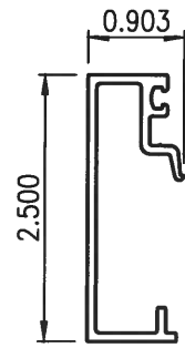
18 SUN-8214 FACE CAP Scale: 6" = 1'-0"
