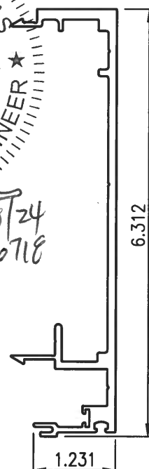
28 SUN-8210 B.G. SPLIT MULLION Scale: 6" = 1'-0"
