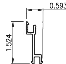
32 SUN-7053 CORNER FC CLIP Scale: 6" = 1'-0"
