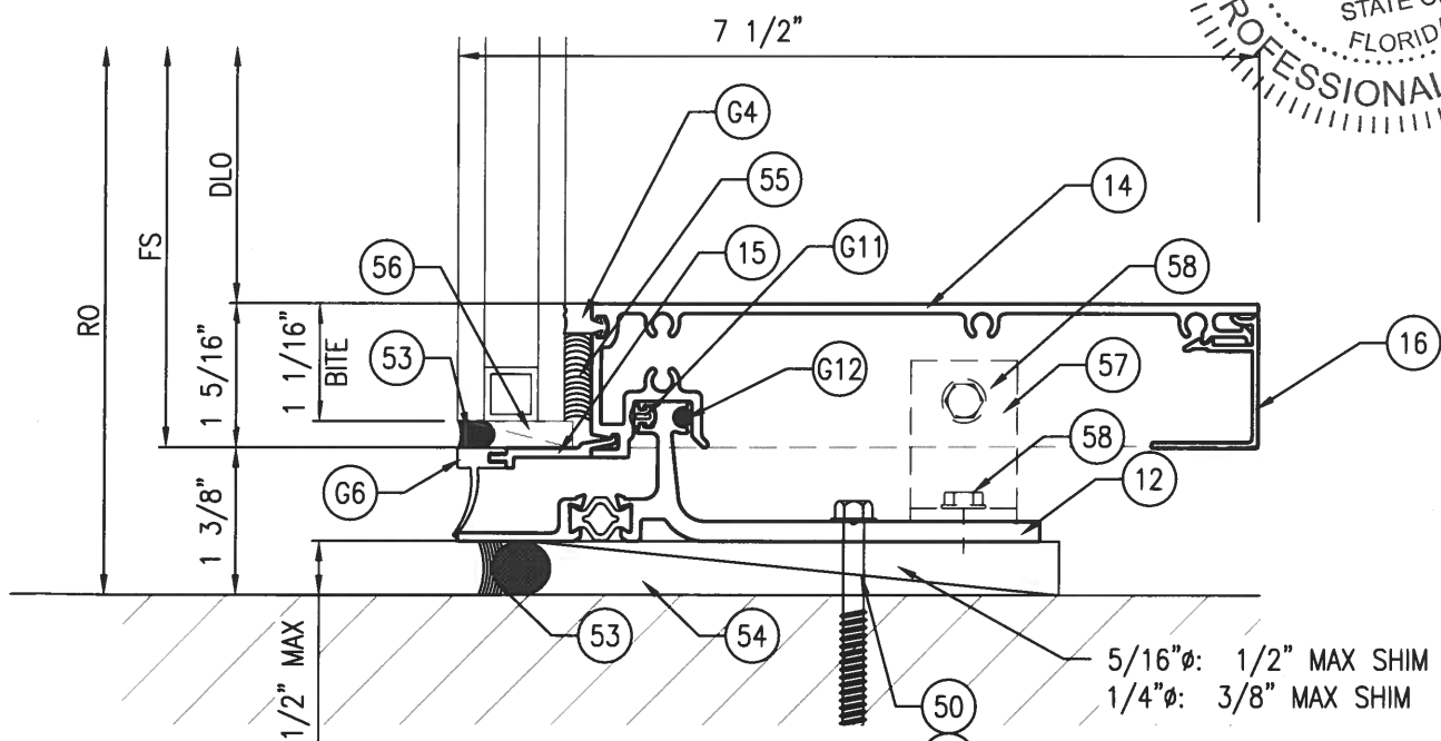
1 SUN 800T SILL SSG Scale: 6" = 1'-0"
