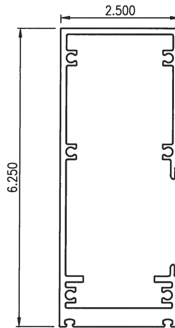
26 SUN-8213 B.G. JAMB Scale: 6" = 1'-0"
