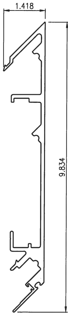
24 SUN-8150 90° SPLIT MULLION Scale: 6" = 1'-0"
