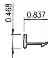
30 SUN-6132 MULLION CLIP Scale: 6" = 1'-0"
