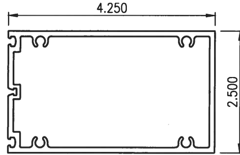
20 SUN-6122 HORIZONTAL Scale: 6" = 1'-0"
