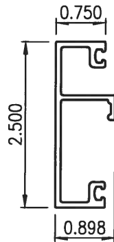
19 SUN-6315 FACE CAP Scale: 6" = 1'-0"
